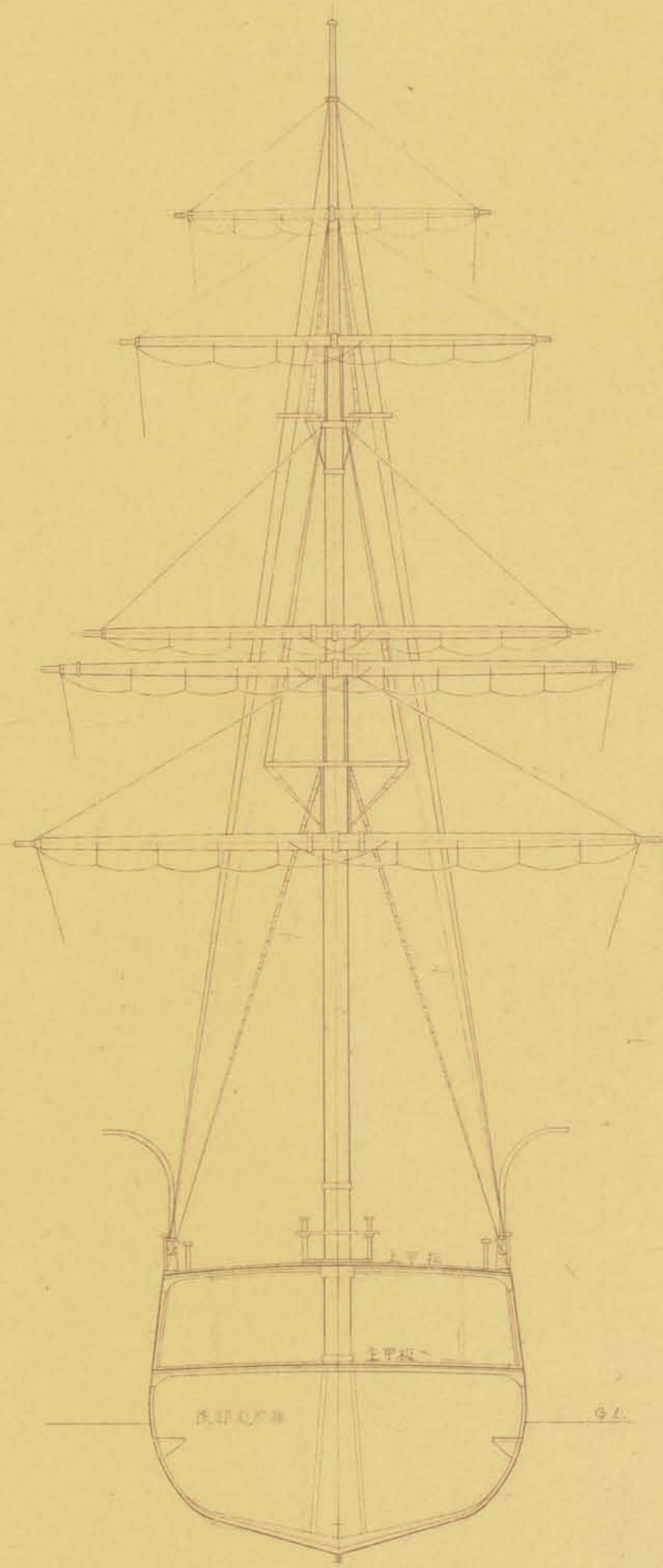
メインマスト横断面図
